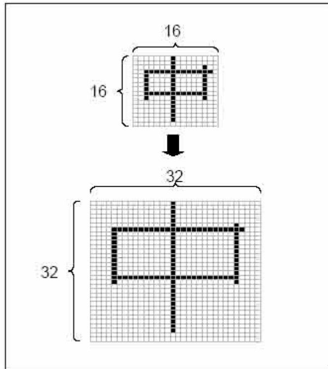
图5-16: 字型放大
