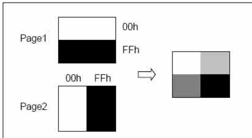
图 5-18: 灰阶
