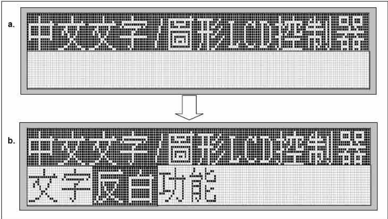
图 5-10: 反白显示
