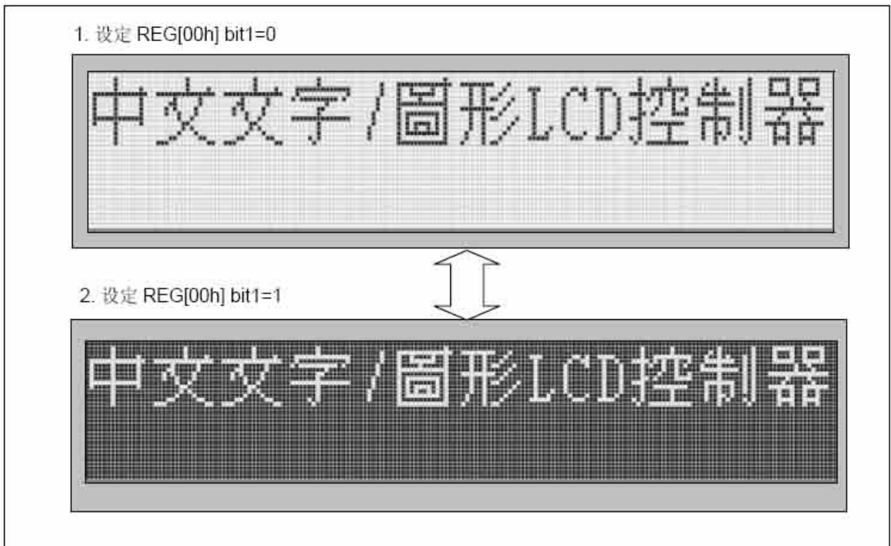
图 5-9: 屏幕闪烁
